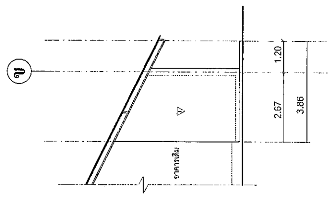
รูปด้าน 2 ขนาดส่วน 1:50
