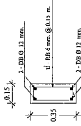
GB SECTION ก, ก'
